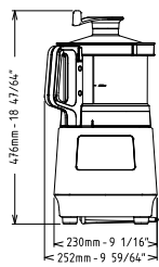
Zij aanzicht
